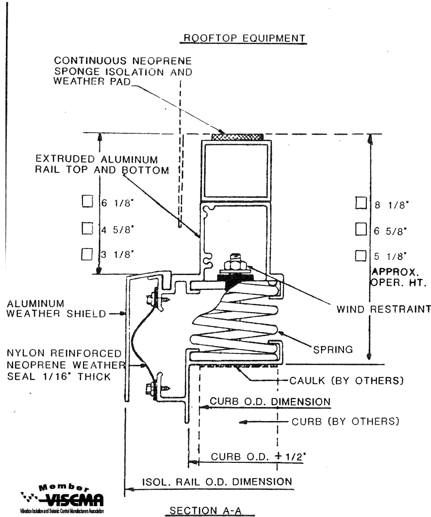
SECTION A-A
